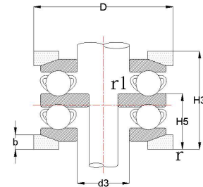
調心座金付
