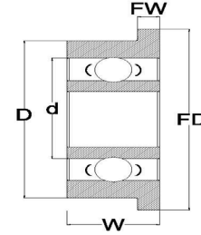
凸緣型
