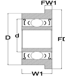
凸緣封密型
